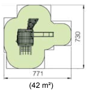
RO533 (sans parcours d'équilibre et sans toit)
