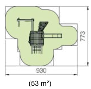
RO532 (avec parcours d'équilibre, sans toit)
